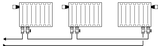
Однокотрубна горизонтальна система опалення
