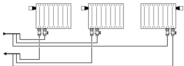
Двотрубна горизонтальна система опалення
